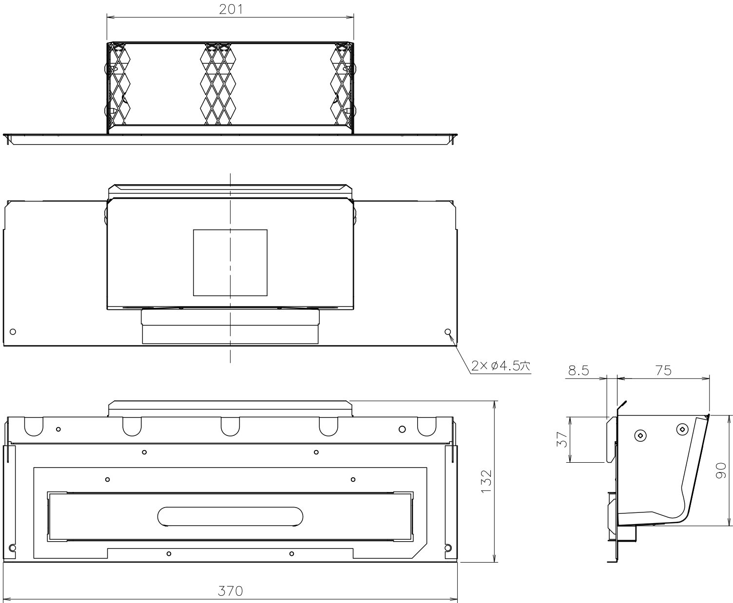
■排気カバー取付板左
