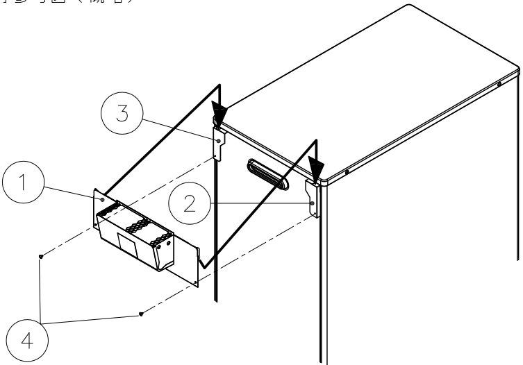
■取付参考図（概略）
