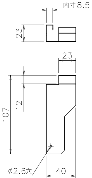
■排気カバー取付板左
