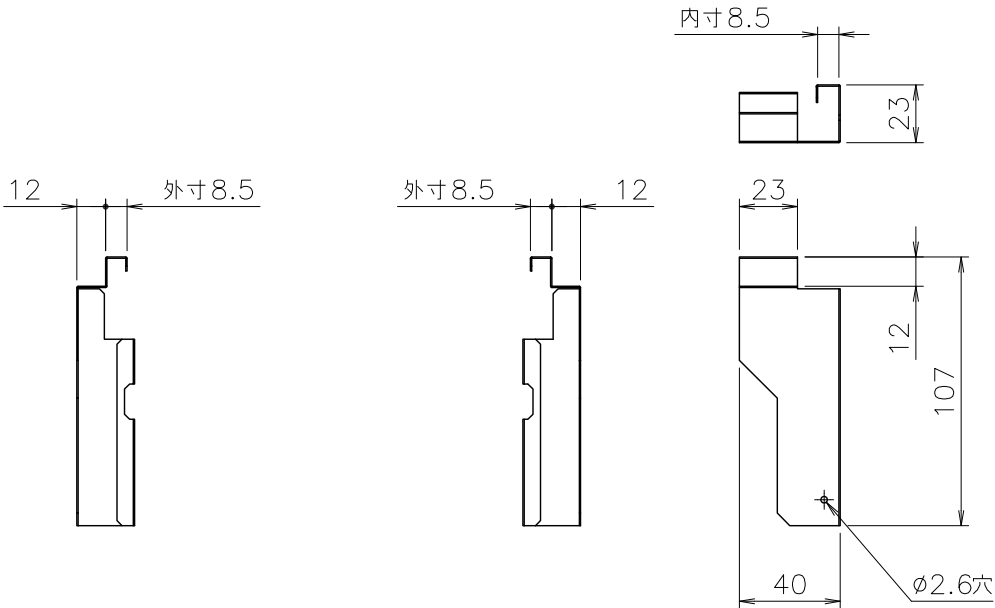
■排気カバー取付板右
