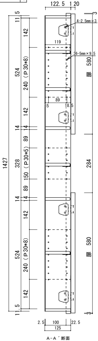
A-A 断面
