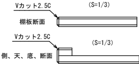
側、天、底、断面
