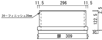
側、天、底、断面
