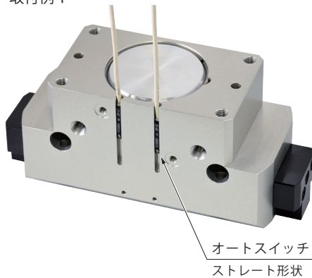
取付例 1
