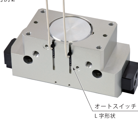
取付例 2
