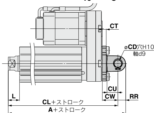
2山クレビス形/LEY 32□□B-□□□D 40 C
