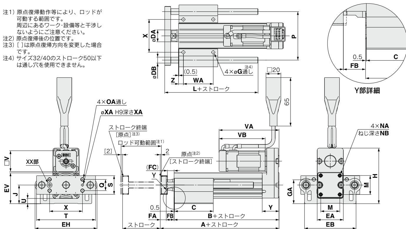
LEYG□M(すべり軸受) [mm]
