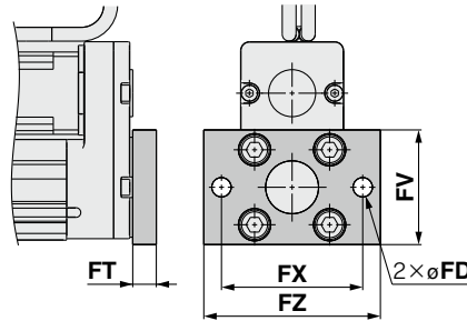
ヘッド側フランジ形/LEY25□□B-□□□G C
