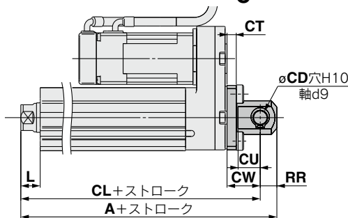
2山クレビス形/LEY 32□□B-□□□D 40 C
