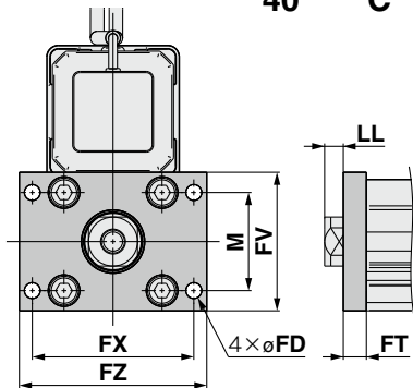
ロッド側フランジ形/LEY 32□□B-□□□F 40 C
