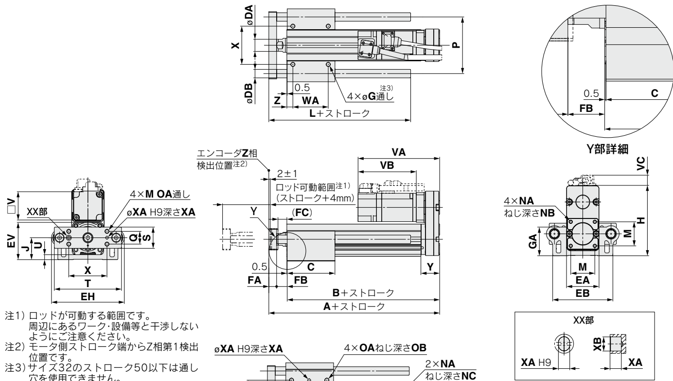
LEYG□L(ボールブッシュ) [mm]
