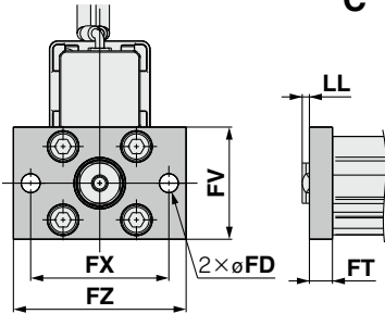
ロッド側フランジ形/LEY 32□□B-□□□F 40 C
