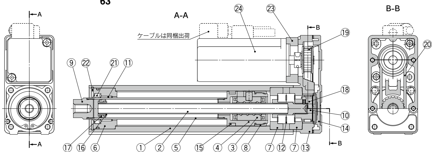
モータ上側折返し／LEY 25 32 63
