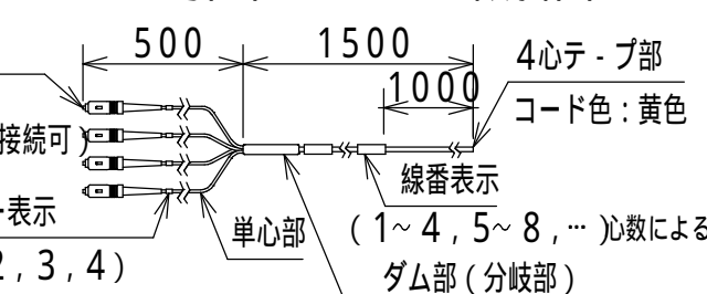
引出しユニット傾斜図
