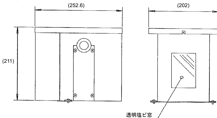
外形図 (mm)
