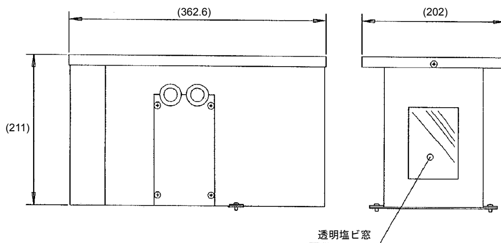
外形寸法図 (mm)
