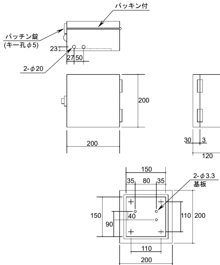
外形寸法図 (mm)
