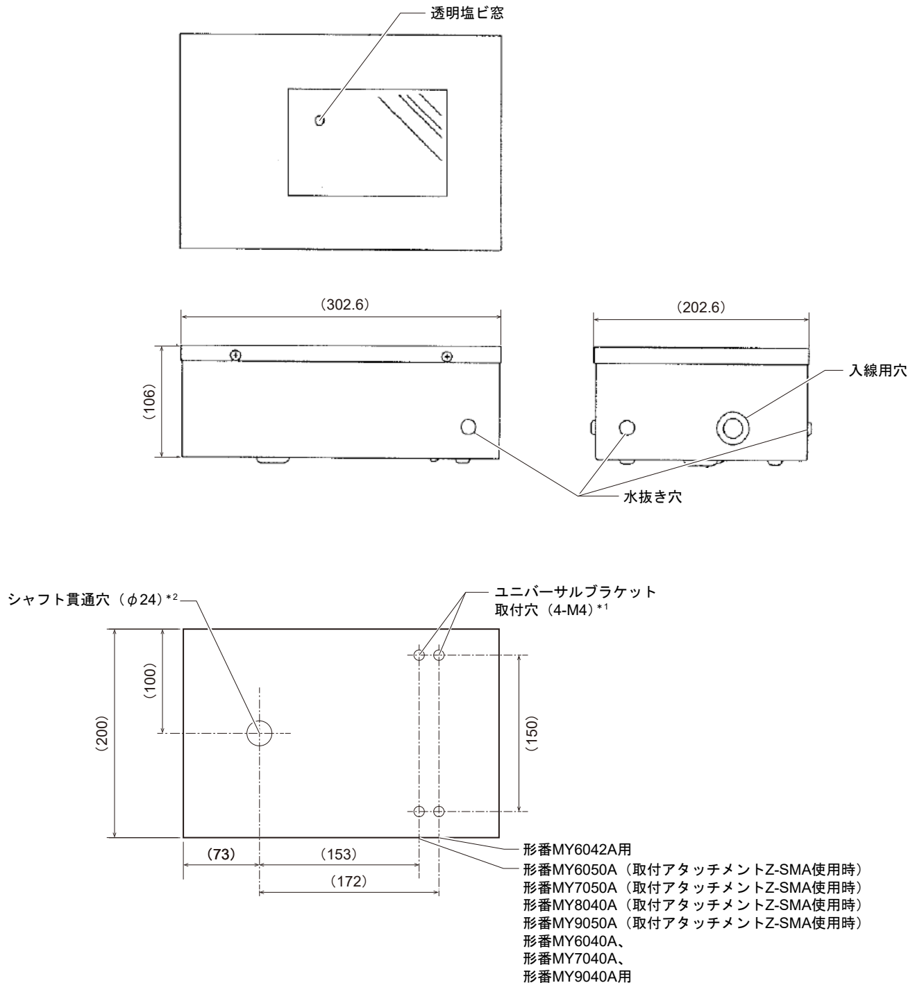
図1 外形寸法図 (単位: mm)
