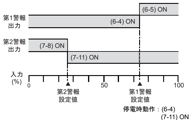
図13 モニタスイッチの動作
