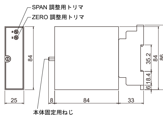
図1 外形寸法図 (本体) (単位：mm)
