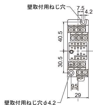
図2 外形寸法図 (専用ソケット) (単位：mm)
