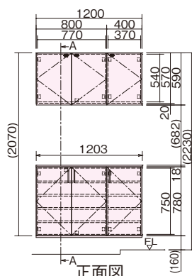
正面図
