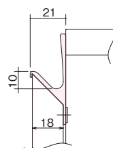
Z部詳細図
