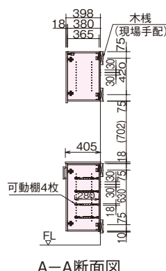
A-A断面図
