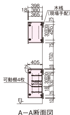
A-A断面図
