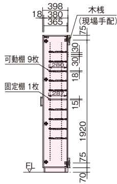
A-A断面図
