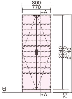
正面図
