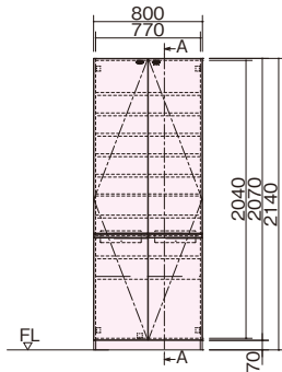
正面図
