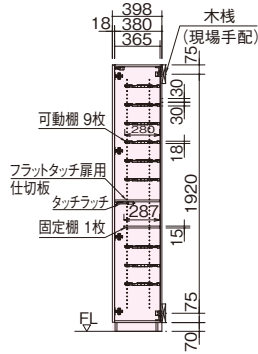
A-A断面図
