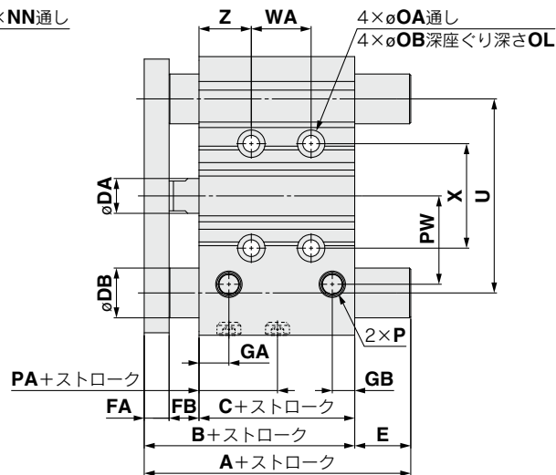
裏面図
