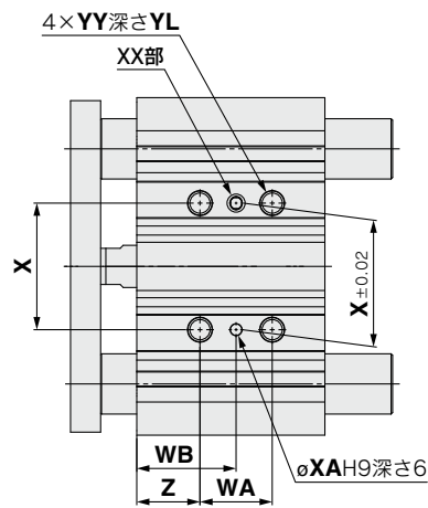
裏面図
