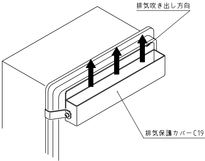
取付完成図 (概略)
