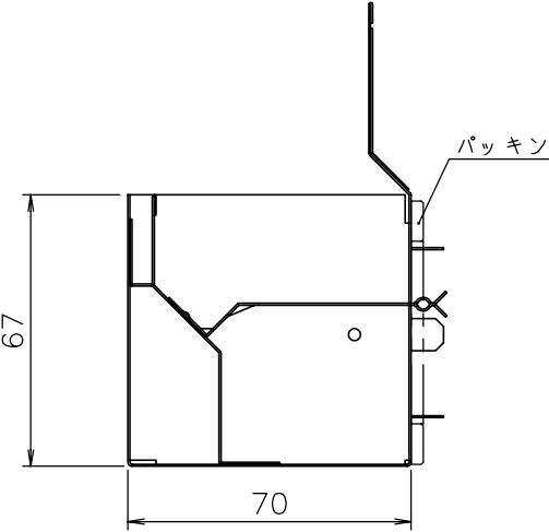
断面 A-A
