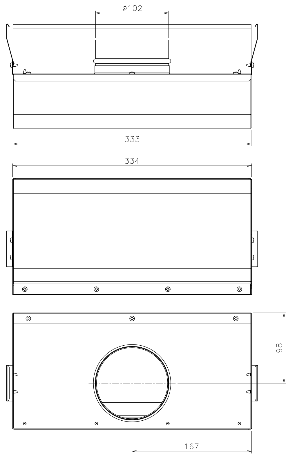
矢視A
