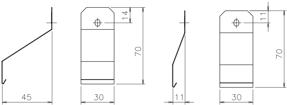
取付板左
