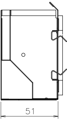
断面A-A
