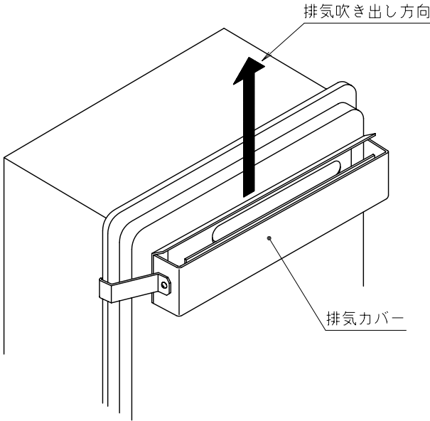
取付完成図（概略）
