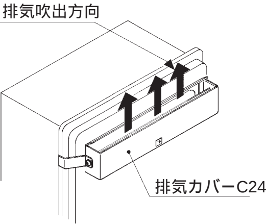
取付完成図（概略）
