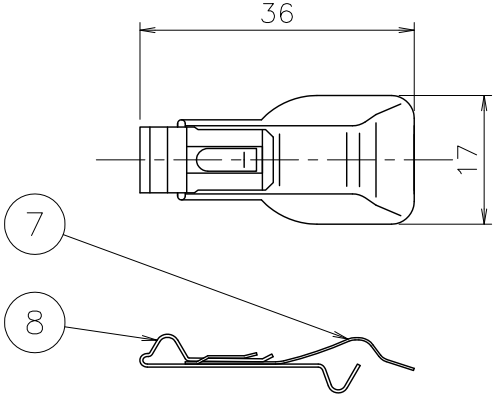
A部詳細 (尺度 1/1)
