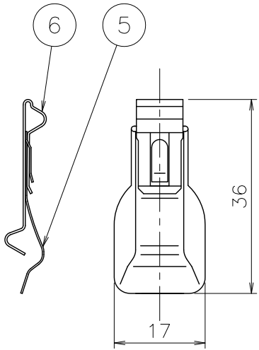
A部詳細（尺度1／1）
