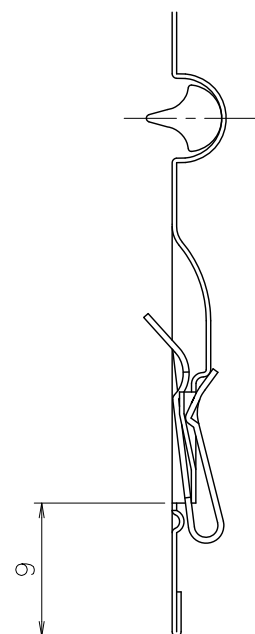
A-A'断面 (S=3:1)
