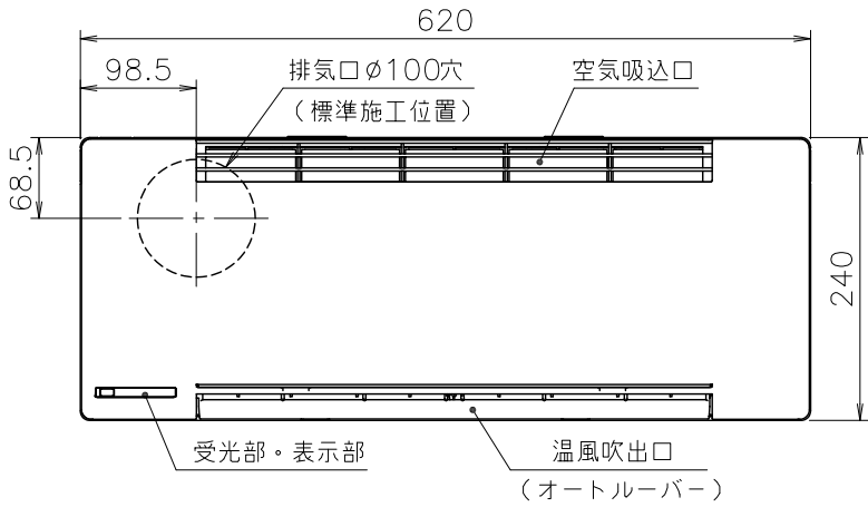
<正面図>
