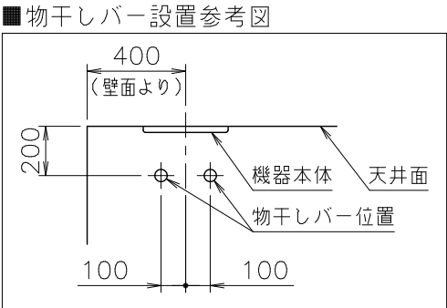
■物干しバー設置参考図
