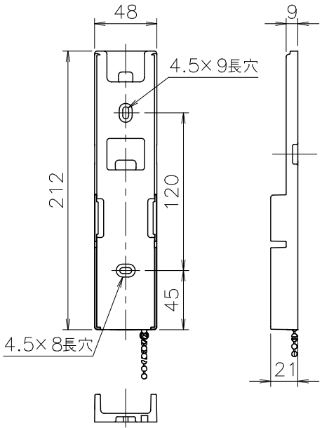
■リモコンホルダー
