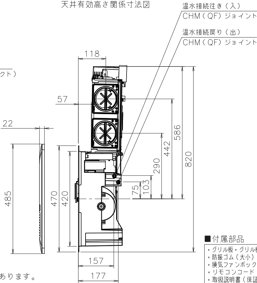
物干しバー収納フック取付 天井有効高さ関係寸法図
