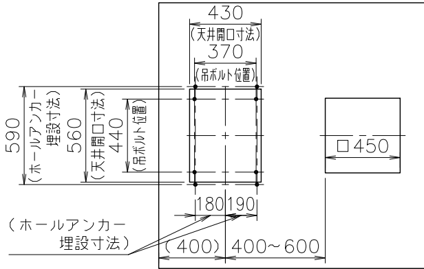
天井開口、吊ボルト、関係寸法図
