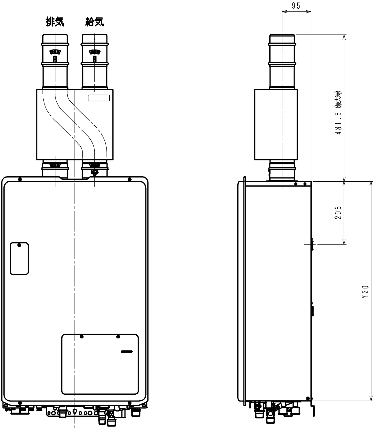
取付図
