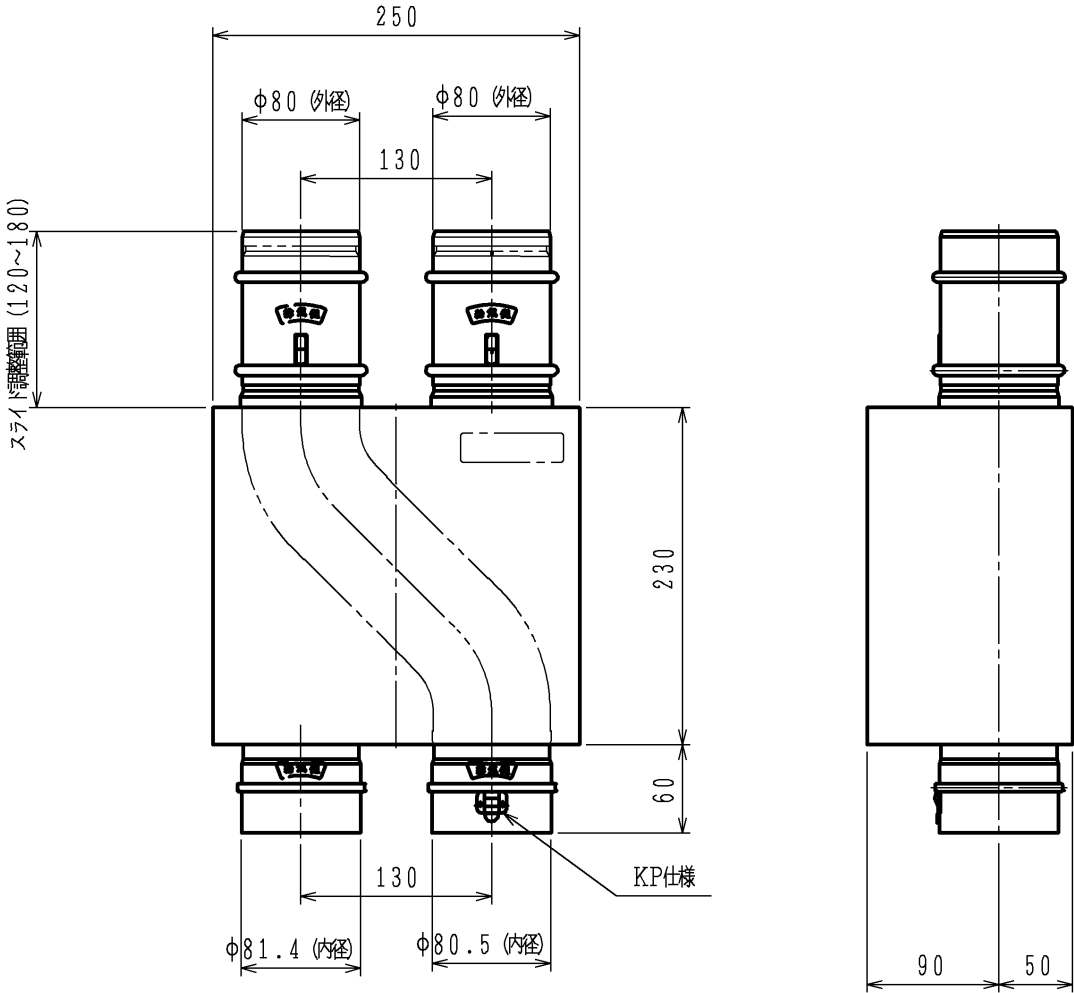
クロスアダプタφ80
