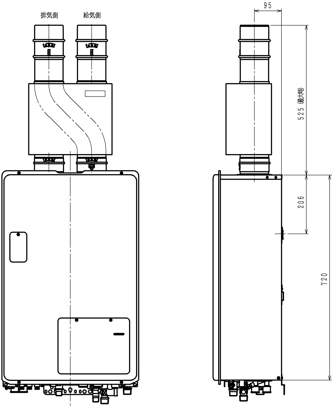
取付図
