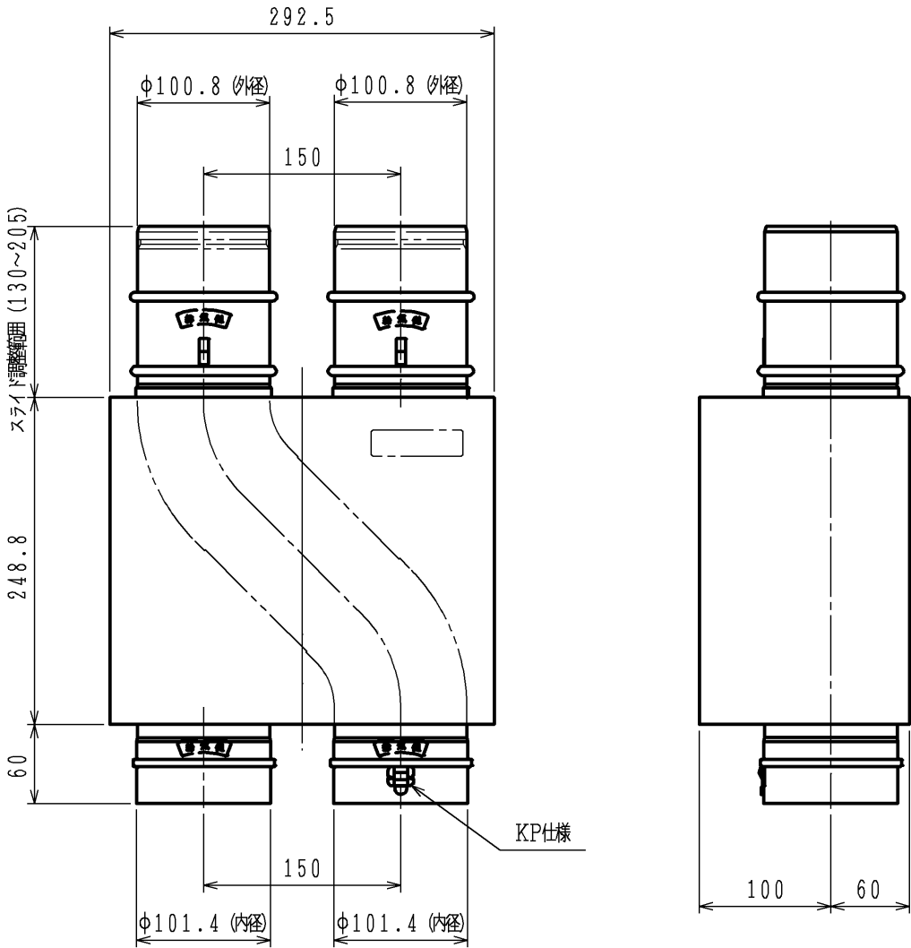
クロスアダプタφ100
