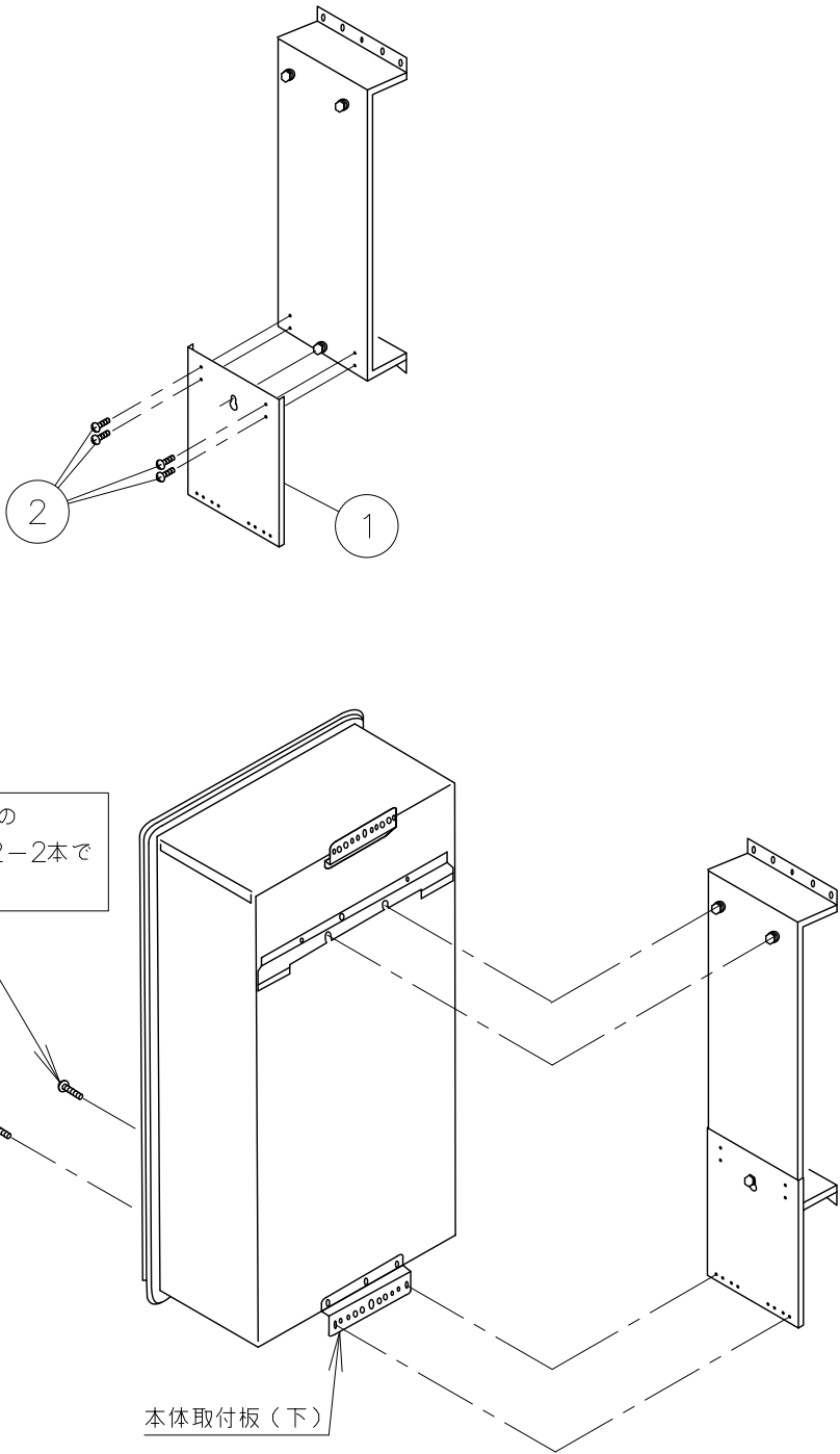
■取付参考図 【壁掛金具FFOA/FT-247・249シリーズの場合】
