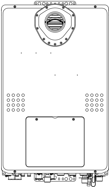
■ 取付参考図（尺度：1／8）
