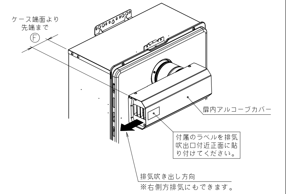
■取り付け参考図
