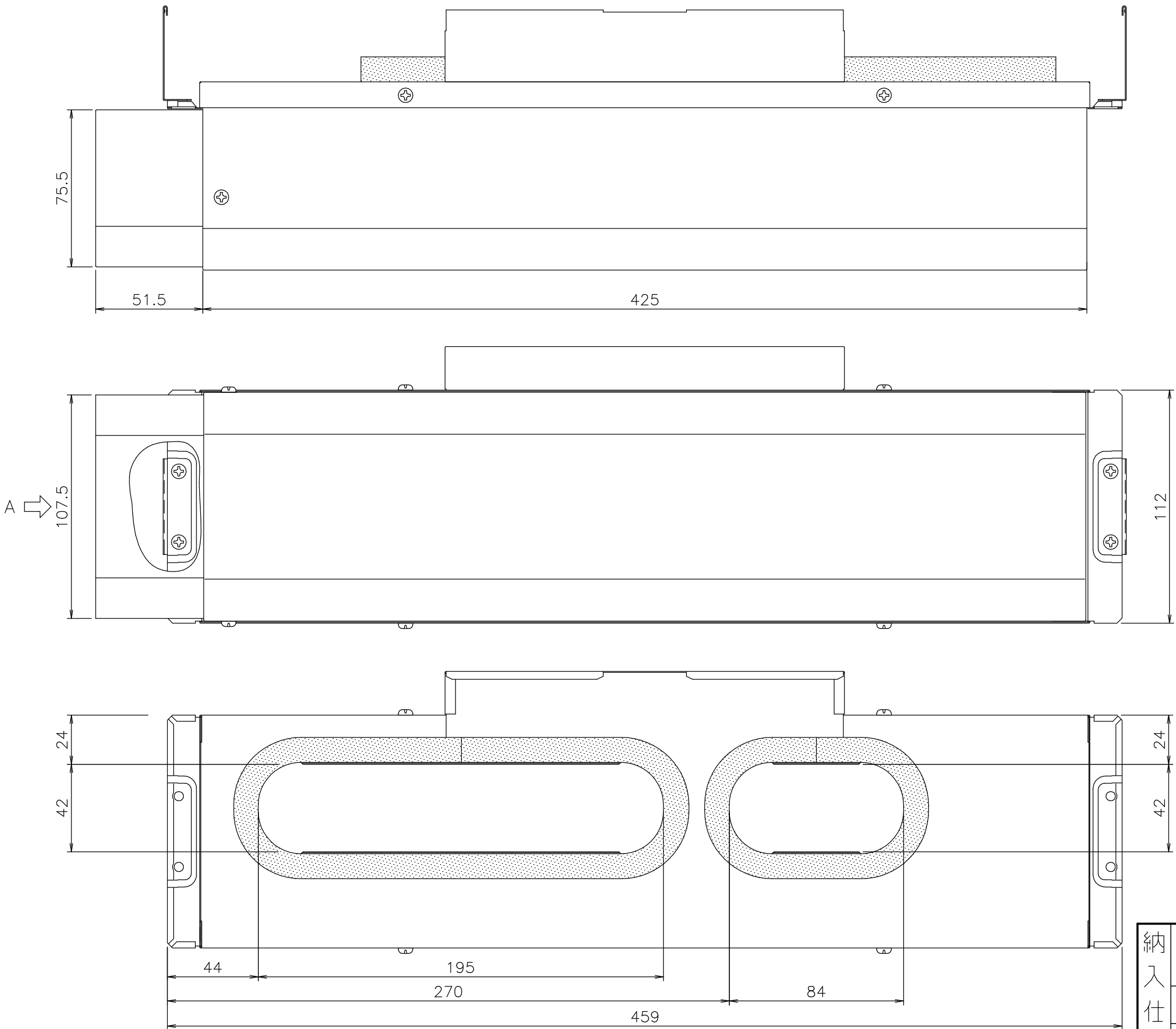
矢視B（排気カバー裏面）
