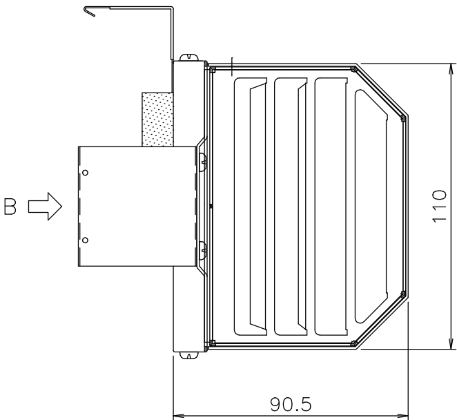
矢視A
