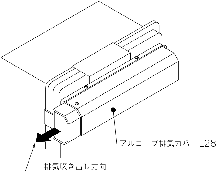
取付完成図（概略）
