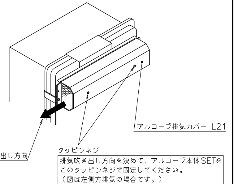
取付完成図（概略）
