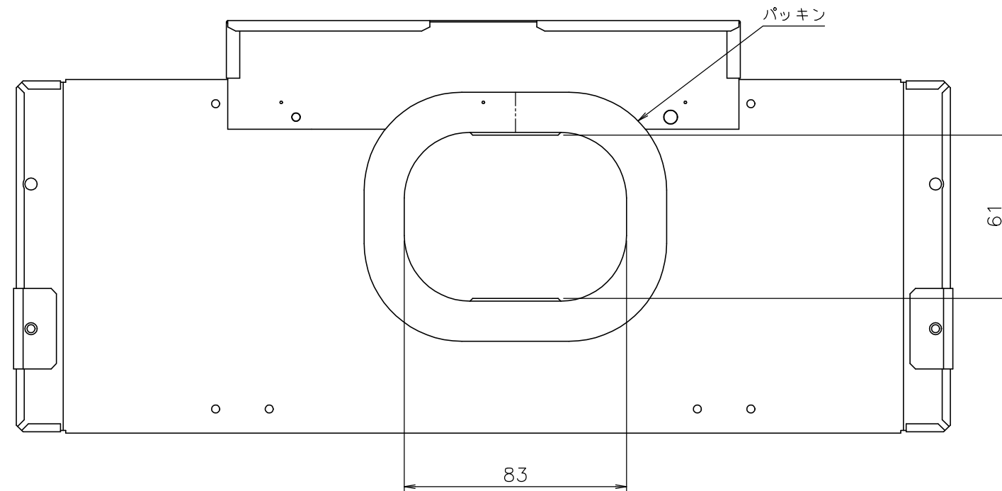
矢視A（排気カバー裏面）
