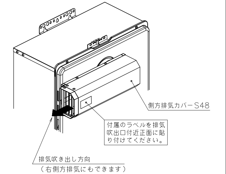
■ 取り付け参考図 1
