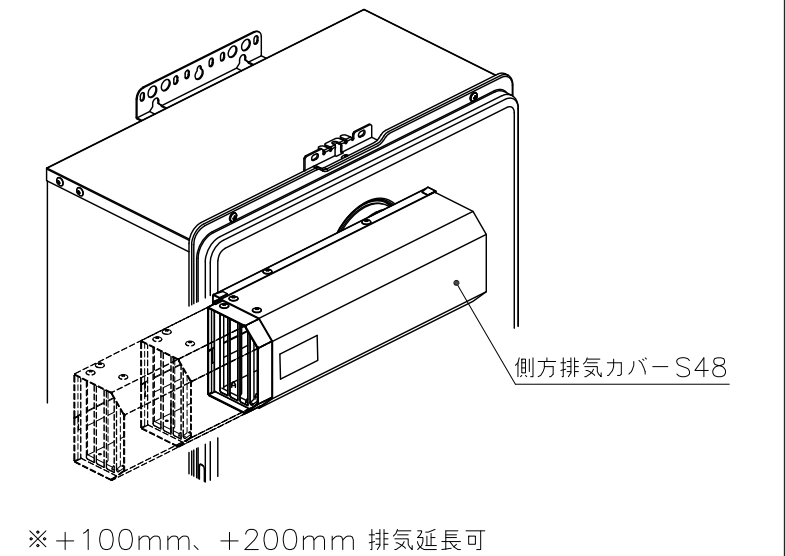
■ 取り付け参考図 2
