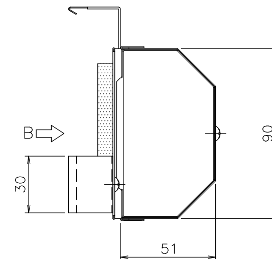
矢視A（排気アダプタ側面）
