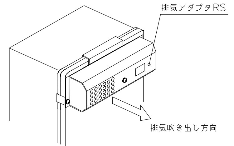
取付完了図（概略）
