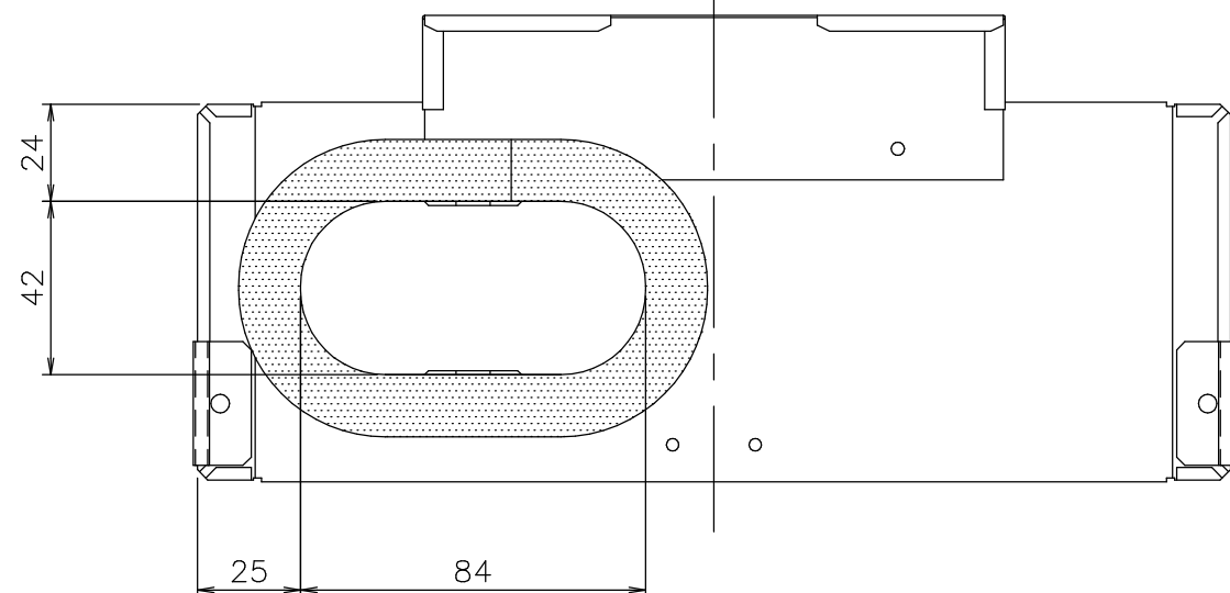
矢視B（排気アダプタ裏面）
