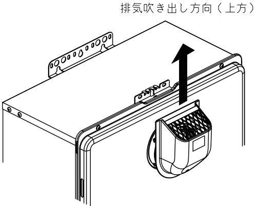
■ 取り付け参考図
