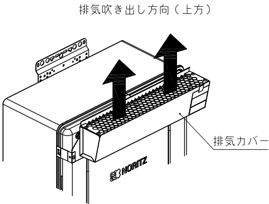
■取り付け参考図
