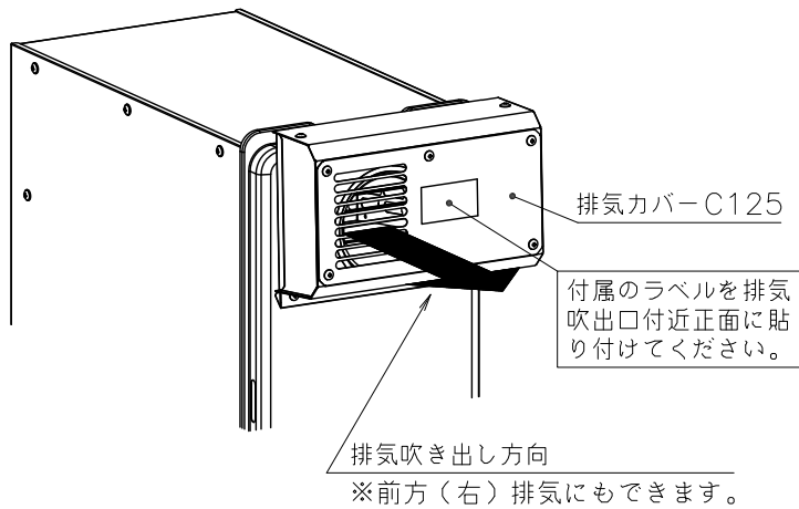
■ 取り付け参考図
