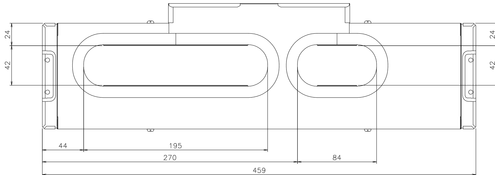
矢視A（排気カバー裏面）
