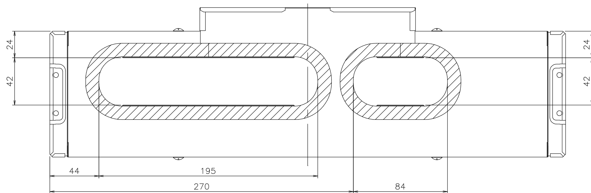
矢視A (排気カバー裏面)
