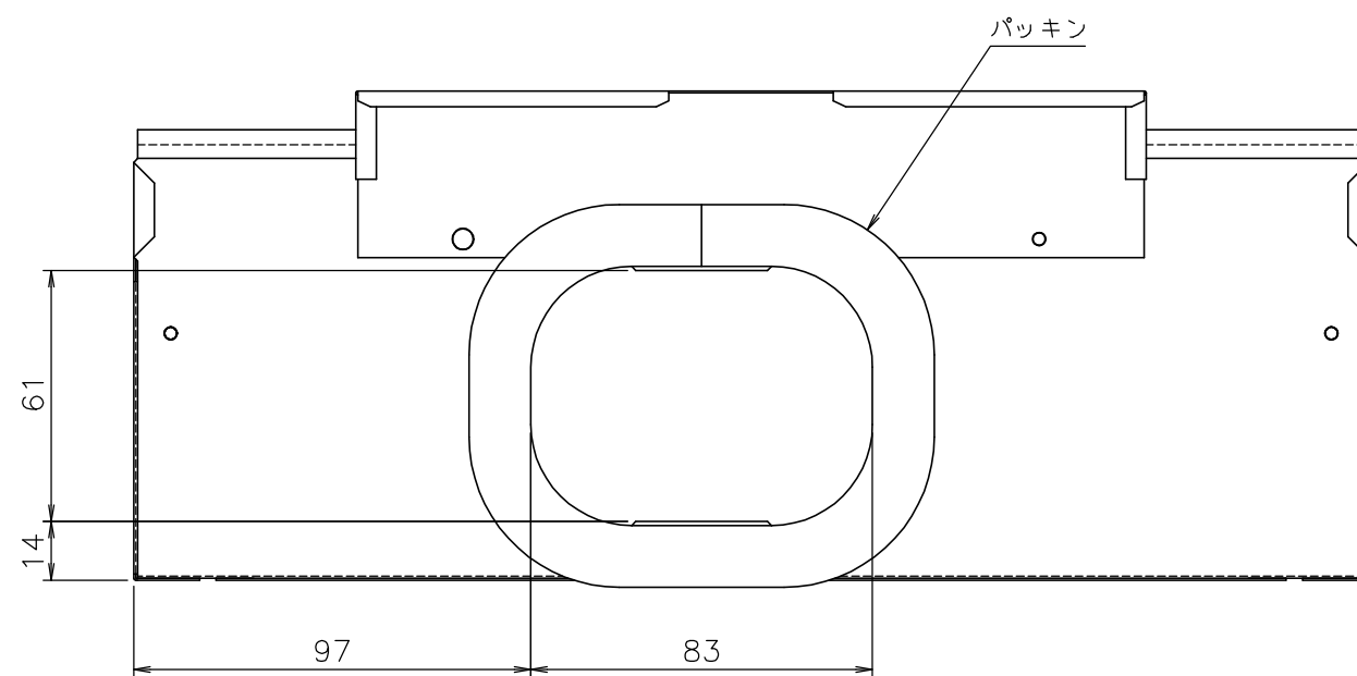
矢視A（排気カバー裏面）
