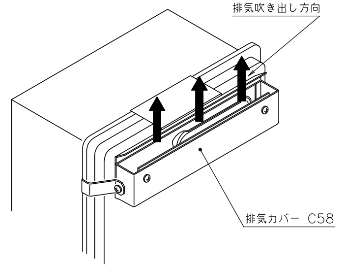
取付完成図（概略）
