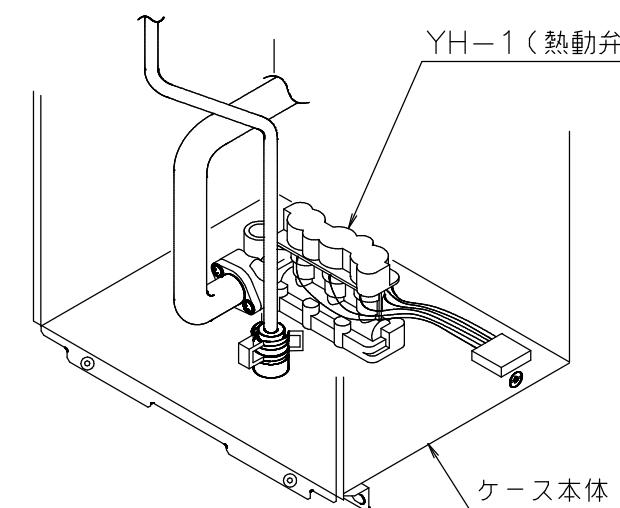
取付要領図（概略）
