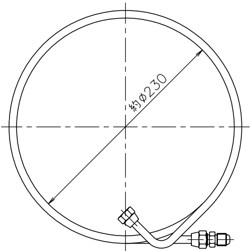
納入形態（尺度1／4）
