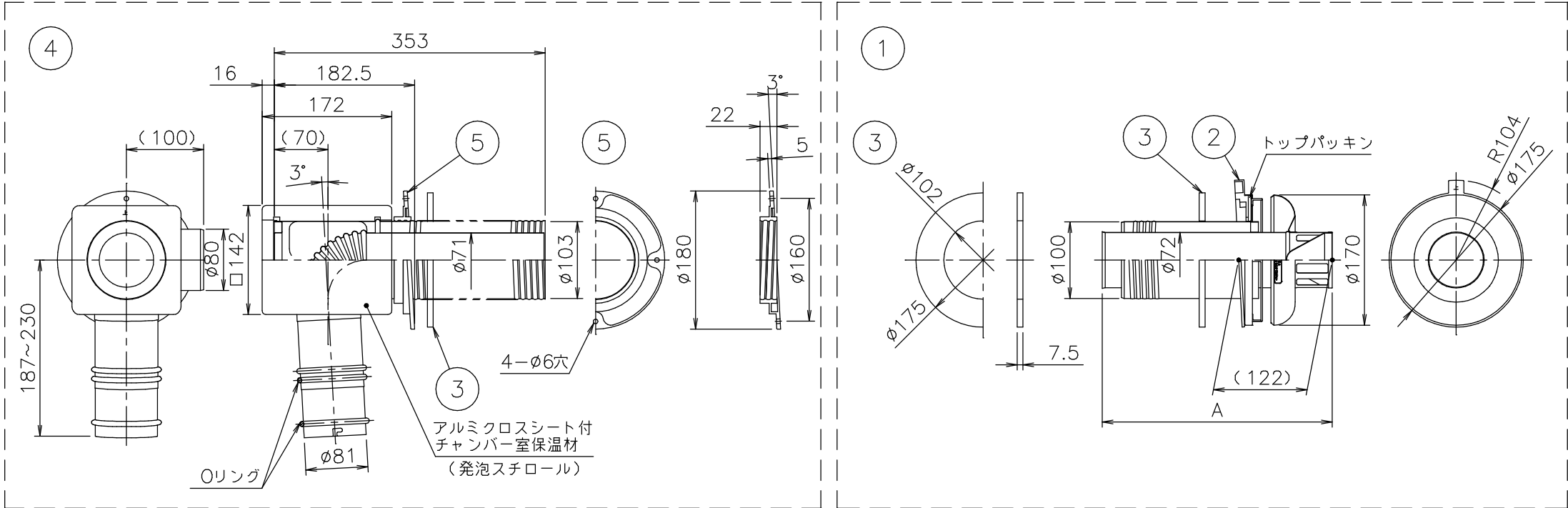
背面図
