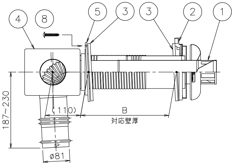
側面図
