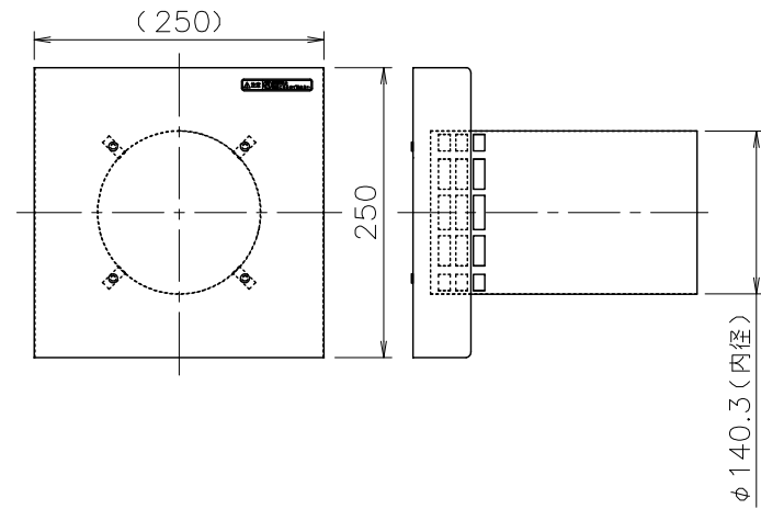
③丸ダクトA：1本
