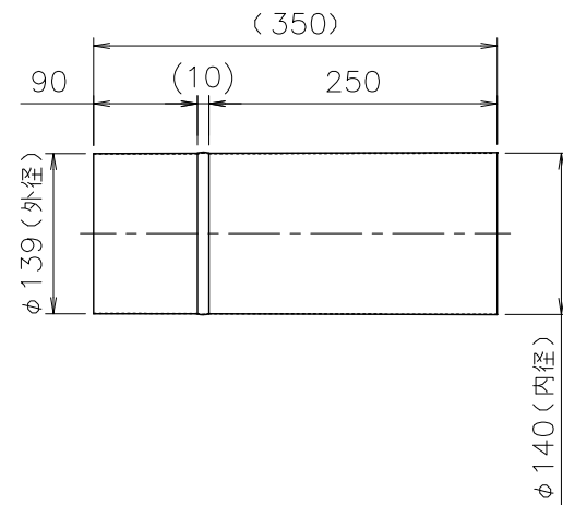
③丸ダクトA：1本
