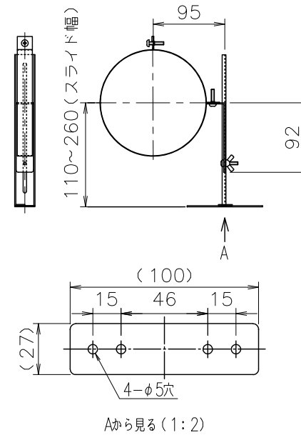
⑤固定金具：2組
