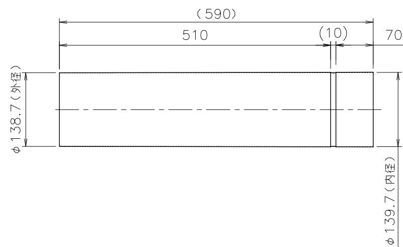
④丸ダクトB：2本
