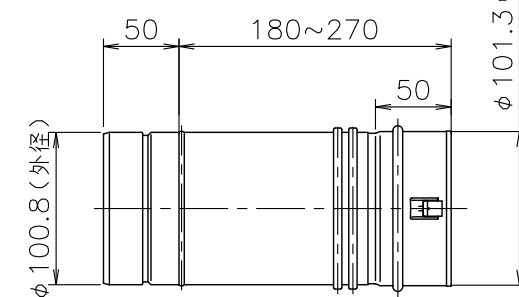
③φ100KPスライド管200型
