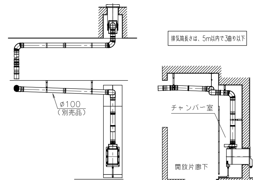
同一風圧帯での排気延長仕様
