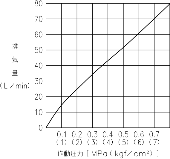
■排気P-Q特性
