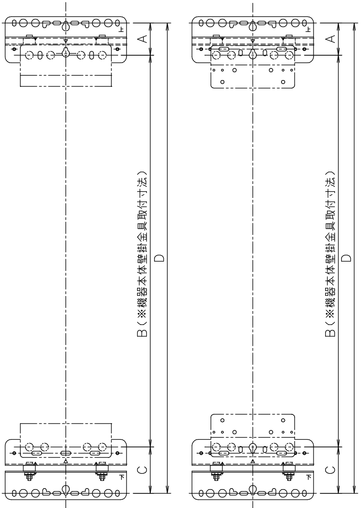
■取付要領図（尺度1/4） （取付例 GH-1210W） ■取付要領図（尺度1/4） （取付例 GH-712W）
