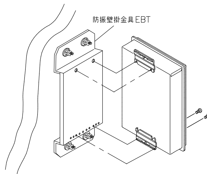
■取付図
