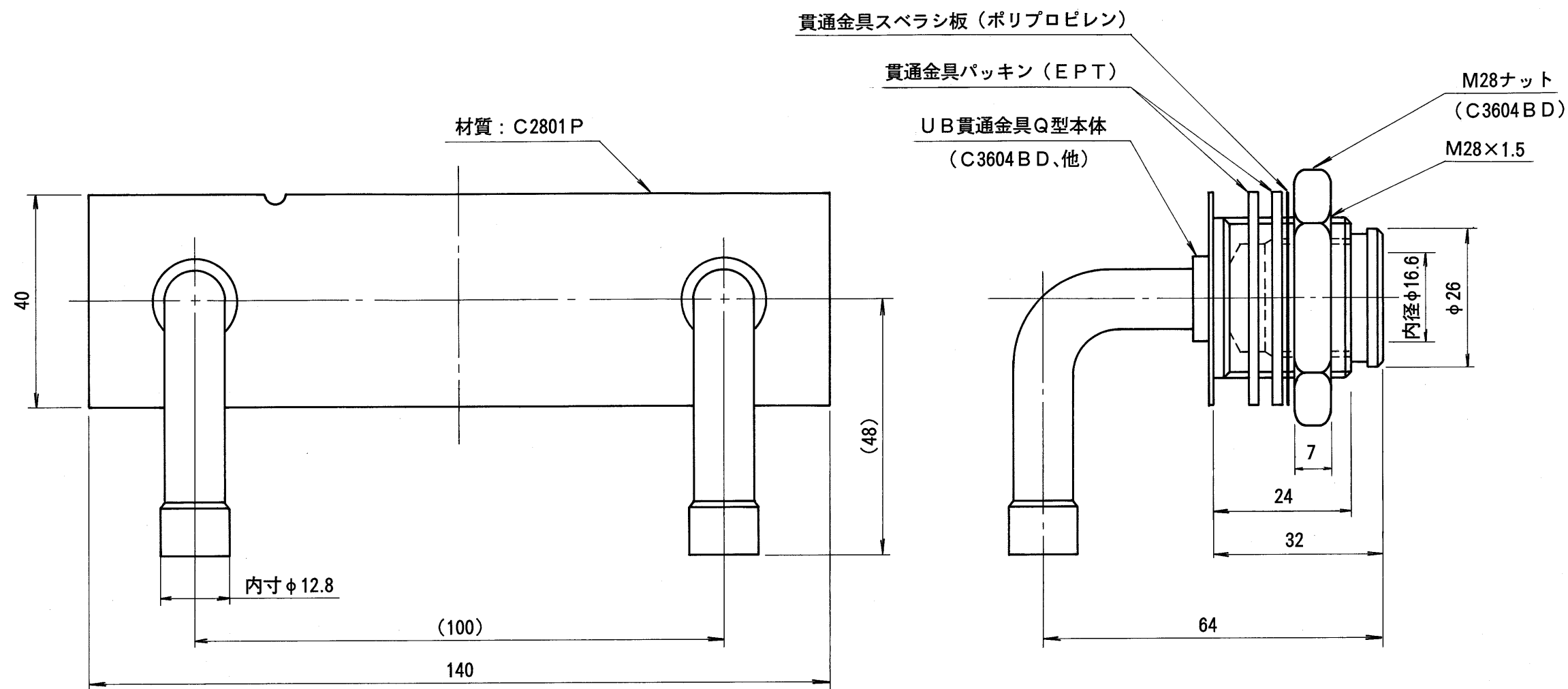
取付図
