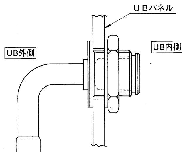
取付図
