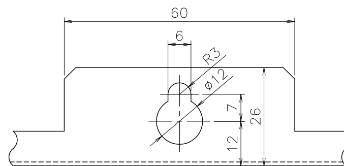
■ A部詳細 (尺度 1/1)
